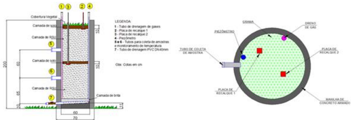
Figura 1 – Corte vertical e planta do aterro experimental
