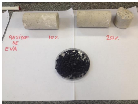
Figura 4 – Tijolo produzido com resíduo: EVA.
